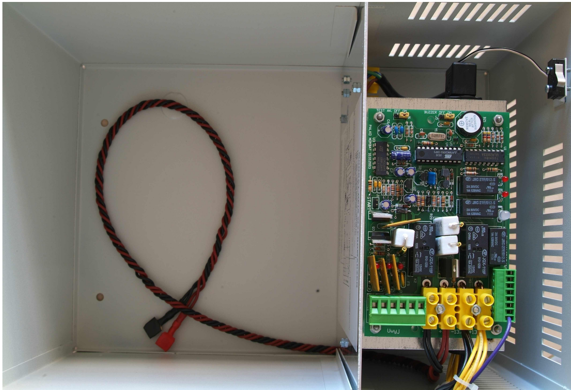
Stacja zasilania STZ1495/38 w obudowie na akumulator 38-44Ah Widok po zdjęciu przedniej osłony. Wymiary 325x230x200
